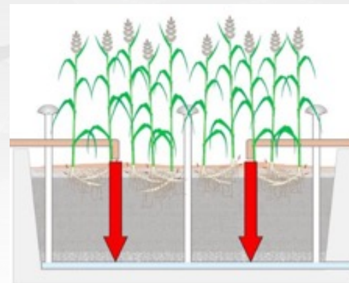
Sous-surfacique à écoulement vertical
