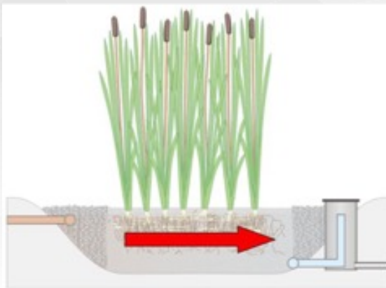
Sous-surfacique à écoulement horizontal
