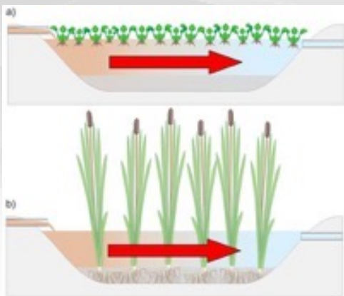
Surfacique à écoulement horizontal
